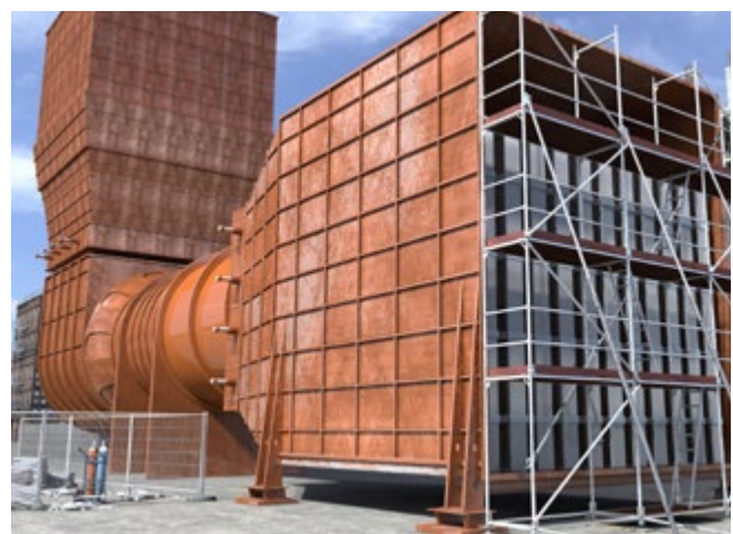
Abb. 153 Schalldämpferkulissen
